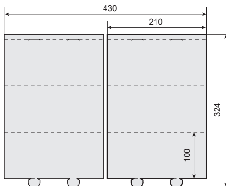
K-25-A3(2)-D-1 430*324
