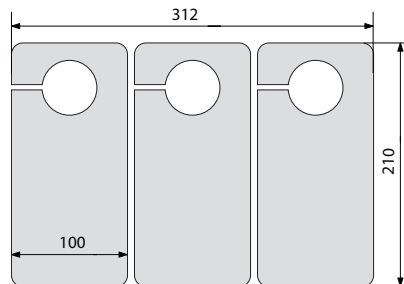
B-38-A4(3)-D-1 312*210
