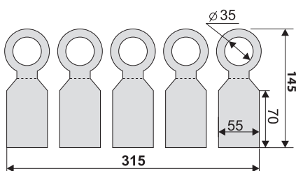
B-32-A4(5)-D-3 145*315
