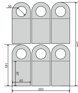
K-228-A4(6)-D-1 203*294
