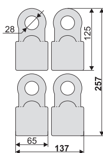
B-34-A4(4)-D-1 137*257
