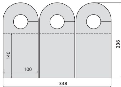
K-103-A4(3)-D-1 338*236
