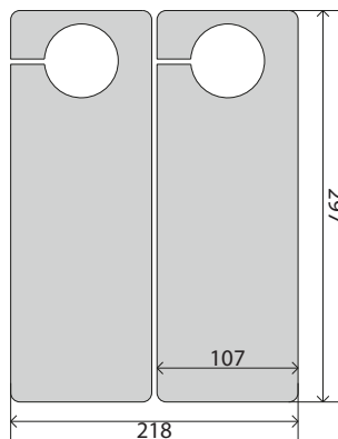
K-226-A4(2)-D-1 218*297
